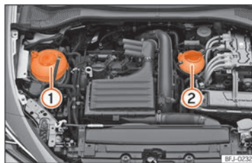
Abb. 234 Motorraum: Kühlmittelbehälter
