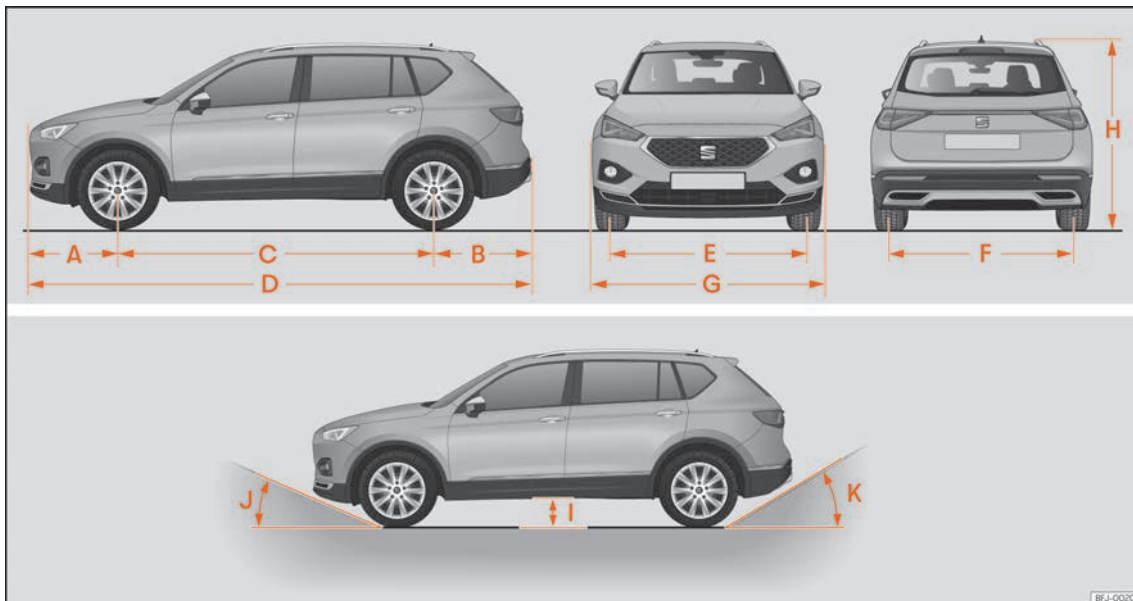
Abb. 259 Abmessungen
