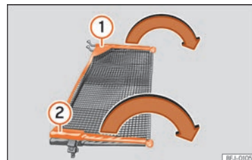
Abb. 131 Netztrennwand ausklappen.
