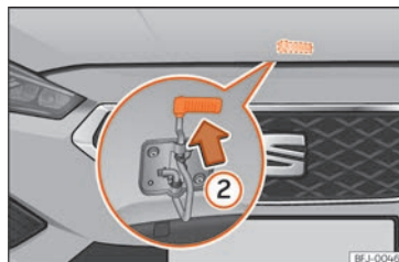
Abb. 240 Hebel unter der Motorraumklappe.
