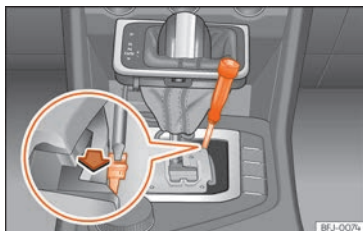
Abb. 172 Wählhebel: Notentriegeln aus der Parkstellung.
