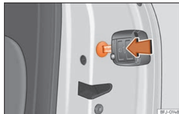
Abb. 82 Notfallsperre der Tür.
