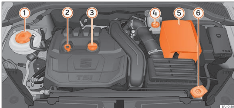
Abb. 241 Abbildung für die Einbaustellen der Elemente
