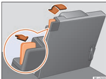
Abb. 122 Dritte Sitzreihe: Sitz in Ladebodenposition klappen.
