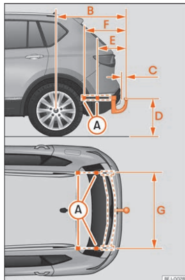
Abb. 222 Maße und Befestigungspunkte für den nachträglichen Einbau einer Anhängervorrichtung
