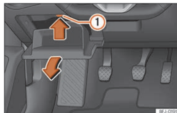
Abb. 49 Auf der Fahrerseite in der Instrumententafel (Linkslenker): Abdeckung des Sicherungskasten.
