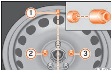
Abb. 36 Radwechsel: Reifenventil (1) und Einbauort der Anti-Diebstahl-Radschraube (2) oder (3).
