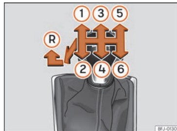
Abb. 168 Schaltschema des 6-Gang-Schaltgetriebes.
