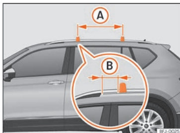
Abb. 134 Befestigungspunkte der Längsträger für den Dachgepäckträger.
