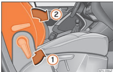
Abb. 109 Beifahrersitz: Sitzlehne nach vorn klappen.
