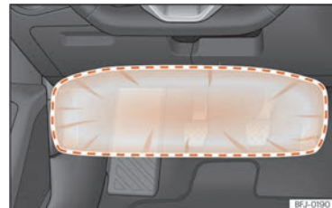
Abb. 20 Auf der Fahrerseite: Wirkungsbereich des Knieairbags.
