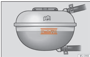
Abb. 225 Im Motorraum: Markierung an dem Motorkühlmittelausgleichsbehälter.
