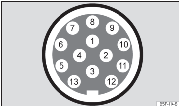
Abb. 214 Schematische Darstellung: Zuweisung der Steckverbindersteife für Anhängerstrom.
