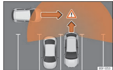
Abb. 193 Schematische Abbildung des Ausparkassistenten: Überwachter Bereich des ausparkenden Fahrzeugs.
