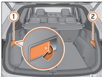
Abb. 112 Im Gepäckraum: Hebel zum Entriegeln des linken Teils ① und des rechten Teils ② der Rücksitzlehne.
