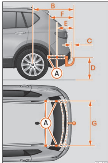
Abb. 216 Maße und Befestigungspunkte für den nachträglichen Einbau einer Anhängervorrichtung
