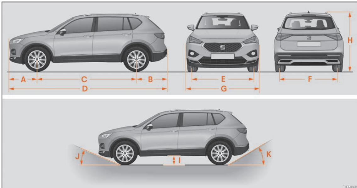
Abb. 236 Abmessungen
