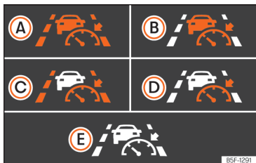
Abb. 187 Am Bildschirm des Kombi-Instruments: Kontrollleuchten.
