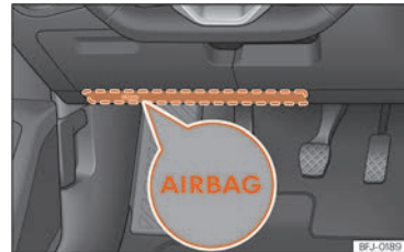
Abb. 19 Auf der Fahrerseite: Einbauort des Knieairbags.
