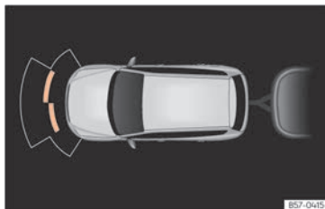
Abb. 205 Bildschirmanzeige der Einparkhilfe im Anhängerbetrieb.
