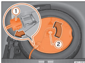
Abb. 235 Im Gepäckraum: Subwoofer ausbauen.
