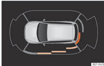
Abb. 204 Anzeige der Einparkhilfe auf dem Bildschirm des Infotainment-Systems.
