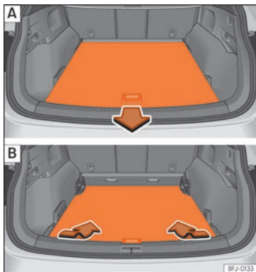
Abb. 121 Im Gepäckraum: Gepäckraumboden in der Höhe verstellen.
