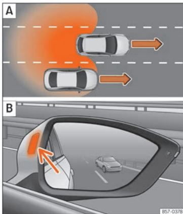
Abb. 192 Schematische Darstellung: A Überholvorgang und anschließender Wechsel auf die rechte Fahrbahn. B Anzeige des Spurwechselassistenten im Außenspiegel rechts.
