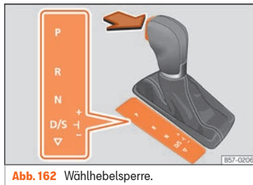
Abb. 162 Wählhebelsperre.
