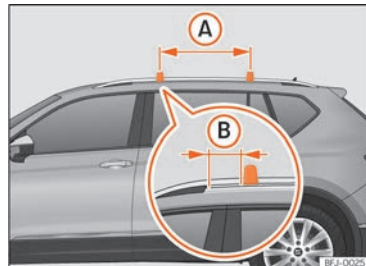
Abb. 130 Befestigungspunkte der Längsträger für den Dachgepäckträger.
