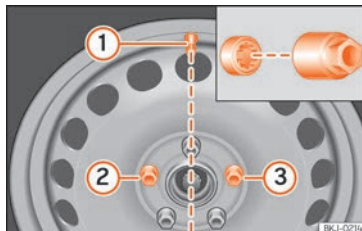
Abb. 39 Radwechsel: Reifenventil ① und Einbauort der Anti-Diebstahl-Radschraube ② oder ③.
