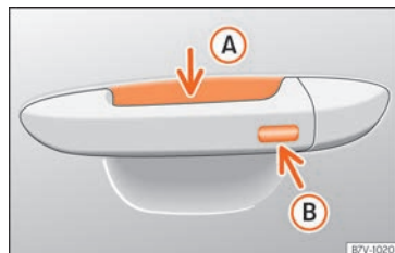
Abb. 100 Türgriff: Sensorflächen
