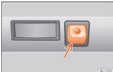
Abb. 295 Im Stoßfänger hinten: Einbaulage der Kamera des Rückfahrassistenten.
