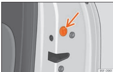
Abb. 103 Notfallsperre der Tür.
