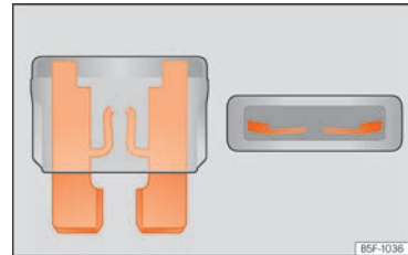
Abb. 69 Darstellung einer durchgebrannten Sicherung.
