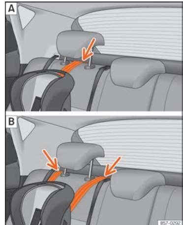
Abb. 40 Befestigungsgurt: korrekte Einstellung und korrekter Einbau
