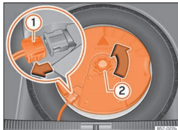
Abb. 318 Im Gepäckraum: Subwoofer ausbauen.
