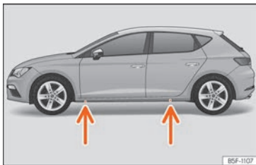
Abb. 78 Querträger: Marken.
