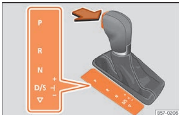
Abb. 258 Wählhebelsperre.
