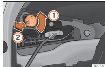
Abb. 120 Lampenhalter ausbauen.
