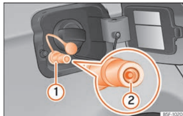
Abb. 262 Geöffnete Tankklappe: Gas-Einfüllstutzen ①, Dichtung des Einfüllstutzens ②.
