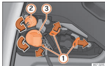
Abb. 202 Lampenhalter ausbauen.
