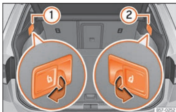
Abb. 81 Im Gepäckraum: Hebel zum Entriegeln der Rücksitzlehne.
