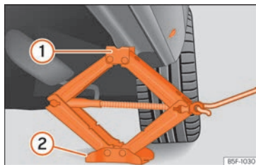
Abb. 225 Längsholm: Wagenheber ansetzen.
