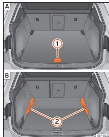
Abb. 169 Variabler Gepäckraumboden: A Hochstellung; B Tiefstellung.
