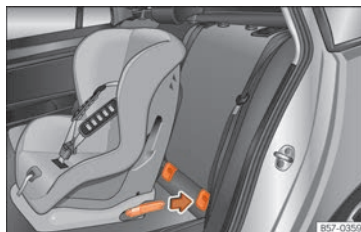
Abb. 40 Rücksitze: Einbau des Kindersitzes mit dem ISOFIX-System.
