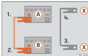
Abb. 192 Anschlusschema für Fahrzeuge mit Start-Stopp-System.
