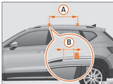
Abb. 178 Befestigungspunkte der Längsträger für den Dachgepäckträger
