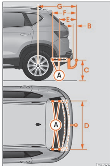
Abb. 183 Maße und Befestigungspunkte für den nachträglichen Einbau einer Anhangervorrichtung
