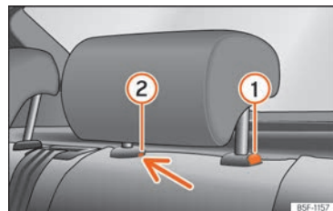
Abb. 78 Kopfstütze hinten: Ausbau.
