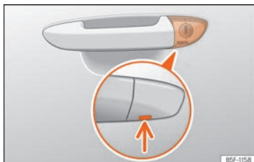
Abb. 55 Fahrertürgriff: verborgener Schließzylinder.
