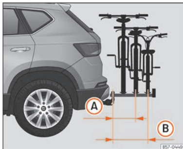
Abb. 182 Schematische Darstellung des maximalen Überstands der Ladung in einem Fahrradträger für zwei oder drei Fahrräder.
