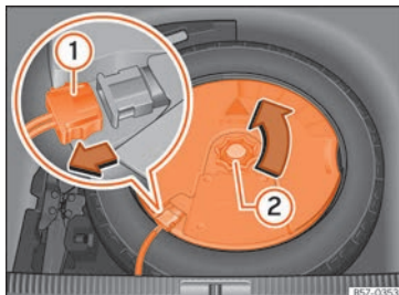
Abb. 223 Im Gepäckraum: Subwoofer ausbauen.
