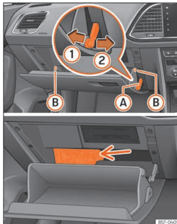
Abb. 50 Handshuhfach (Rechtslenker): Zugang zum Sicherungskasten.
