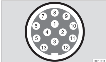
Abb. 201 Schematische Darstellung: Zuweisung der Steckverbindersteife für Anhängerstrom.
