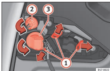
Abb. 113 Lampenhalter ausbauen.
