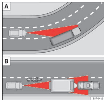
Abb. 190 (A) Fahrzeug in einer Kurve. (B) Vorausfahrender Motorradfahrer außerhalb des Erfassungsbereichs des Radarsensors.
