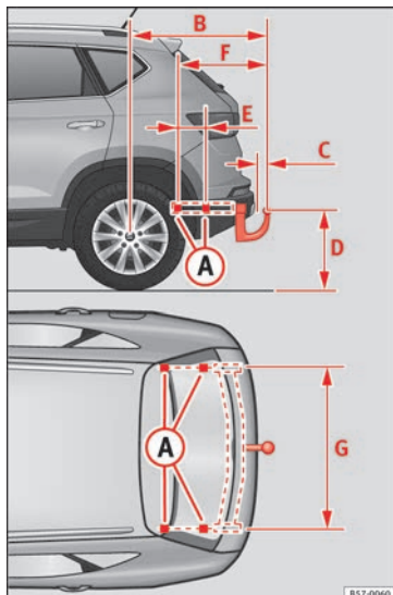
Abb. 232 Maße und Befestigungspunkte für den nachträglichen Einbau einer Anhängervorrichtung
