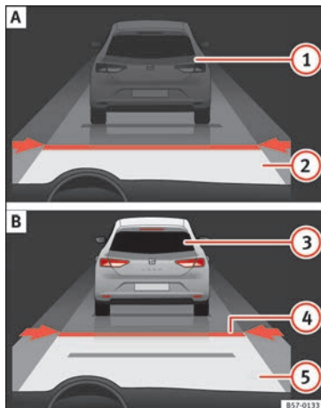
Abb. 184 Im Display des Kombiinstruments: (A) ACC vorübergehend inaktiv, Fahrzeug vor Ihnen erkannt, vorübergehender Abstand eingestellt. (B) ACC aktiv, Fahrzeug vor Ihnen erkannt, ein vorübergehender Abstand wird eingestellt.
