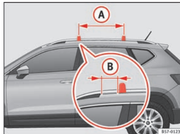
Abb. 166 Befestigungspunkte der Längsträger für den Dachgepäckträger.
