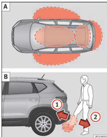
Abb. 127 Schlüsselloses Schließ- und Startsystem Keyless Access: A Näherungsbereiche. B Sensorgesteuertes Öffnen der Gepäckraumklappe (Easy Open).
