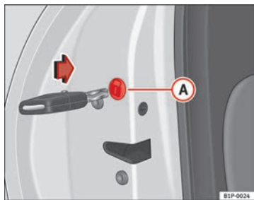
Abb. 60 Notverriegelung der Türen
