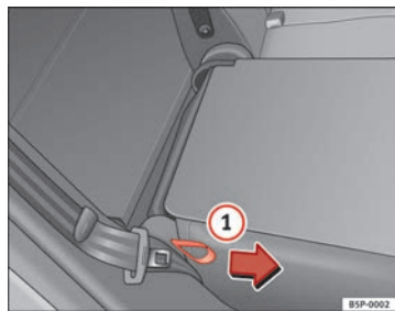
Abb. 100 Umklappen bzw. Aufrechtstellen der Rücksitzlehne
