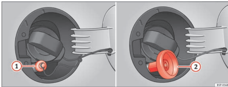
Abb. 161 Geöffnete Tankklappe mit Autogas-Einfillstutzen und Adapter.
