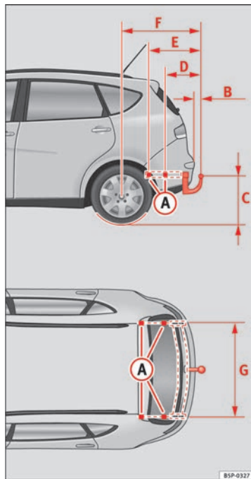
Abb. 159 Befestigungspunkte für die Anhängervorrichtung
