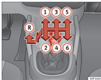
Abb. 144 Ansicht der Mittelkonsole: Schalt-schema eines 6-Gang-Schaltgetriebes
