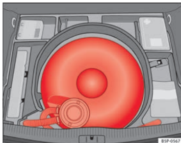
Abb. 162 Autogas-Vorratsbehälter in der Reserveradmulde.
