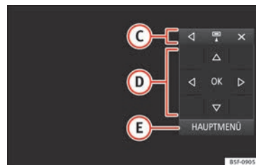
Abb. 39 DVD-Betrieb: Menüsteuerung.
