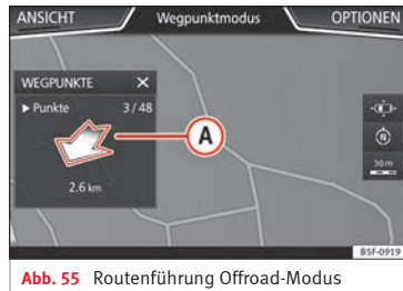
Abb. 55 Routenföhrung Offroad-Modus
