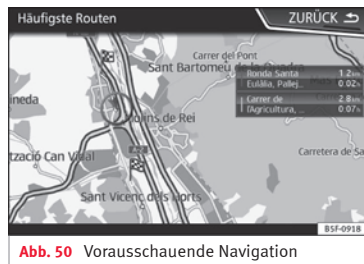
Abb. 50 Vorausschauende Navigation
