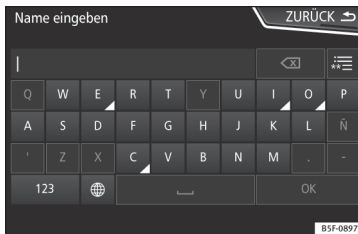
Abb. 71 Suchmaske.
